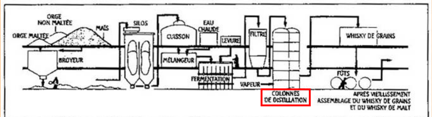
La fabrication des whiskies de grain.
