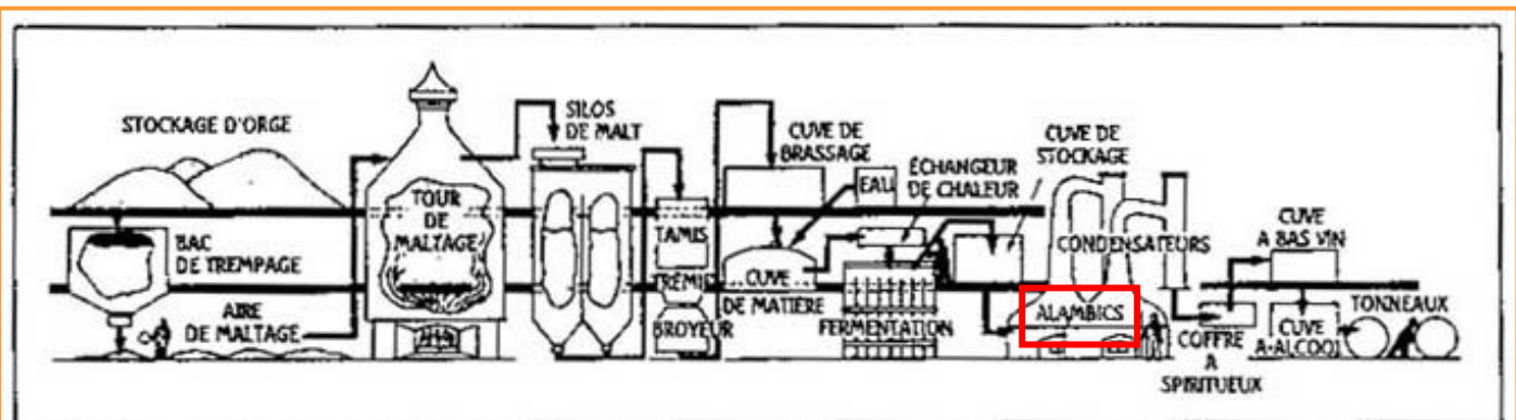
La fabrication des whiskies de malt.
